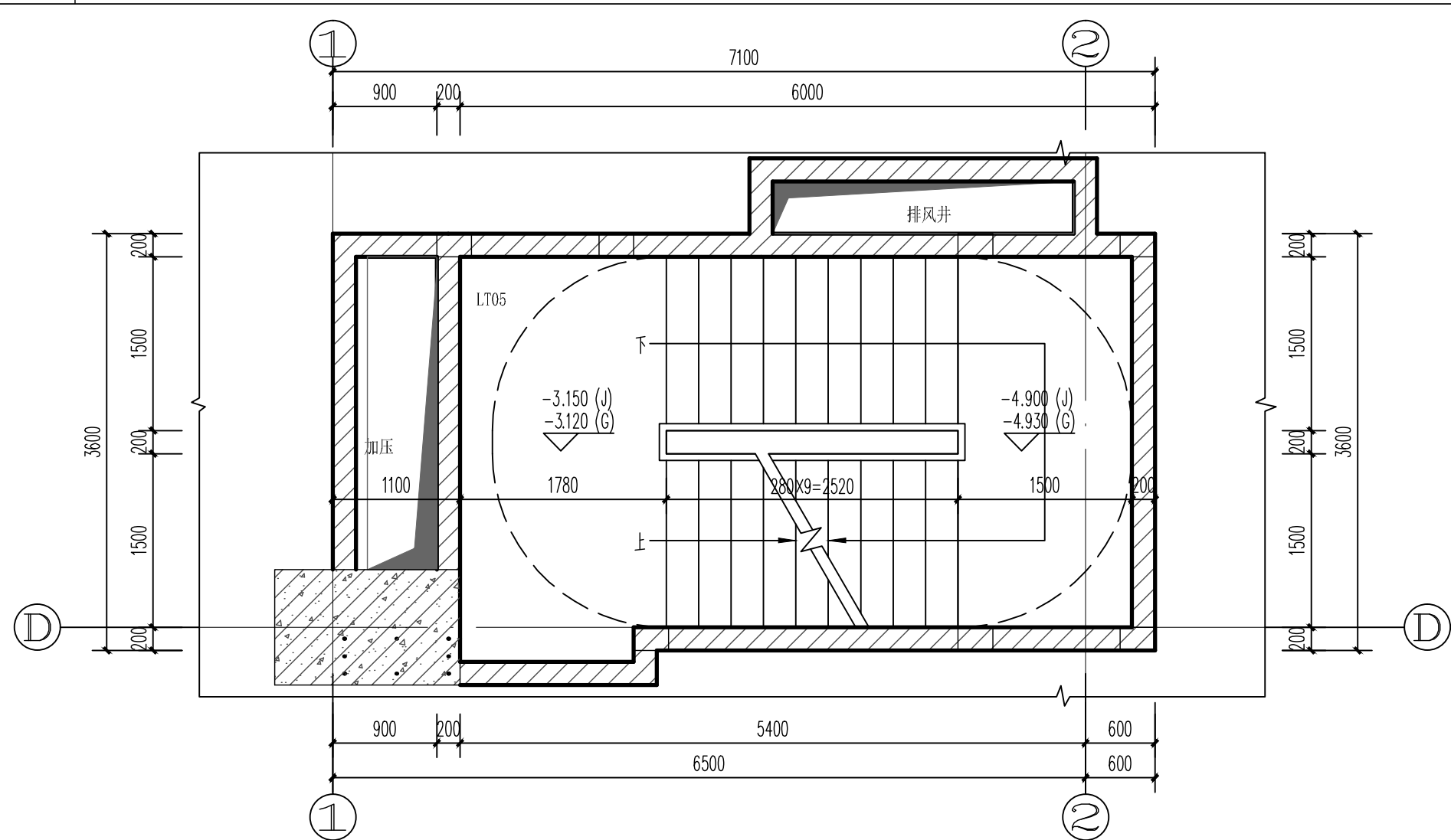
-3.150标高平面
