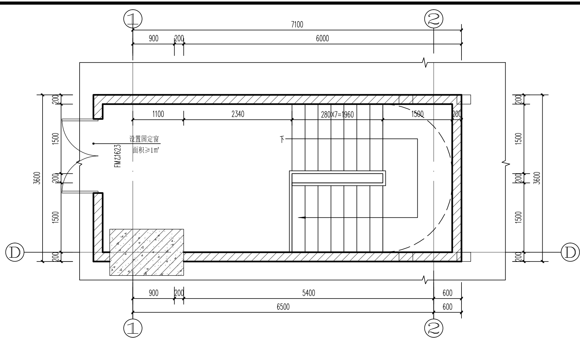
LT05 二层平面
