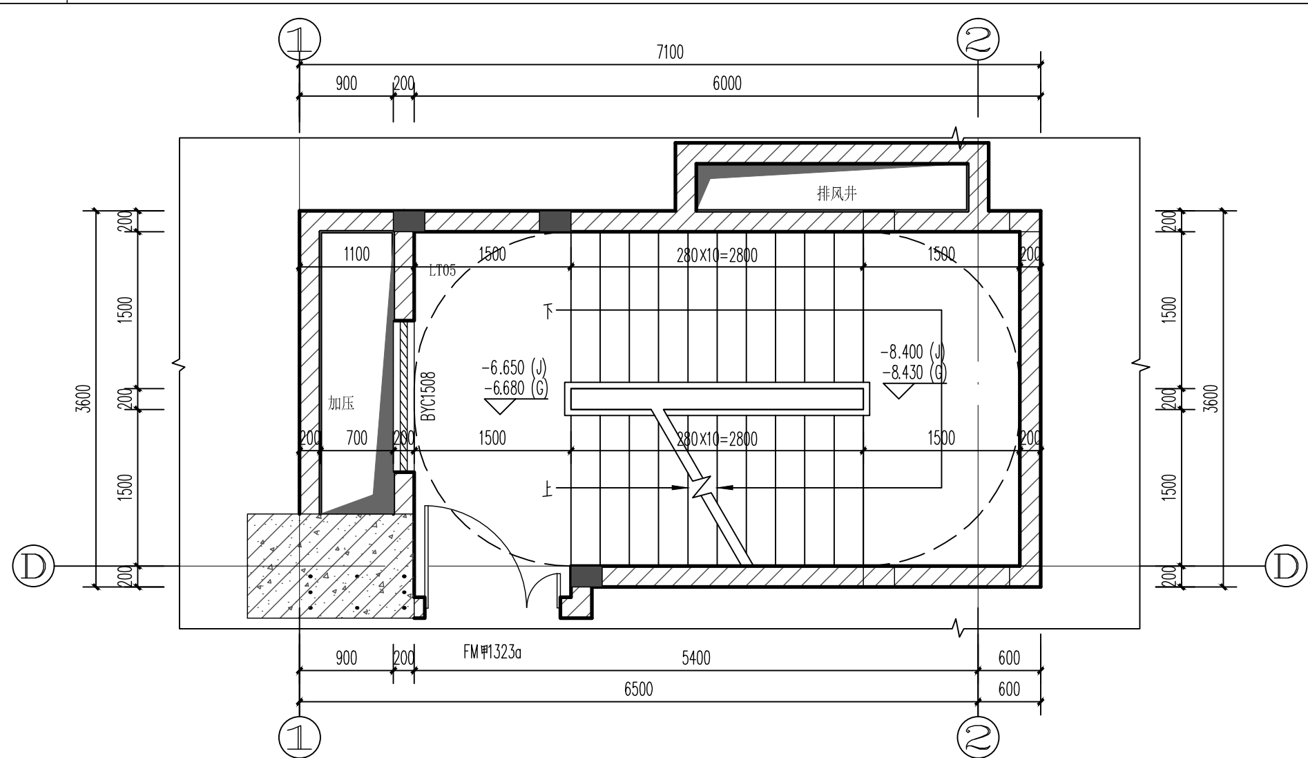
LT05 地下一层平面
