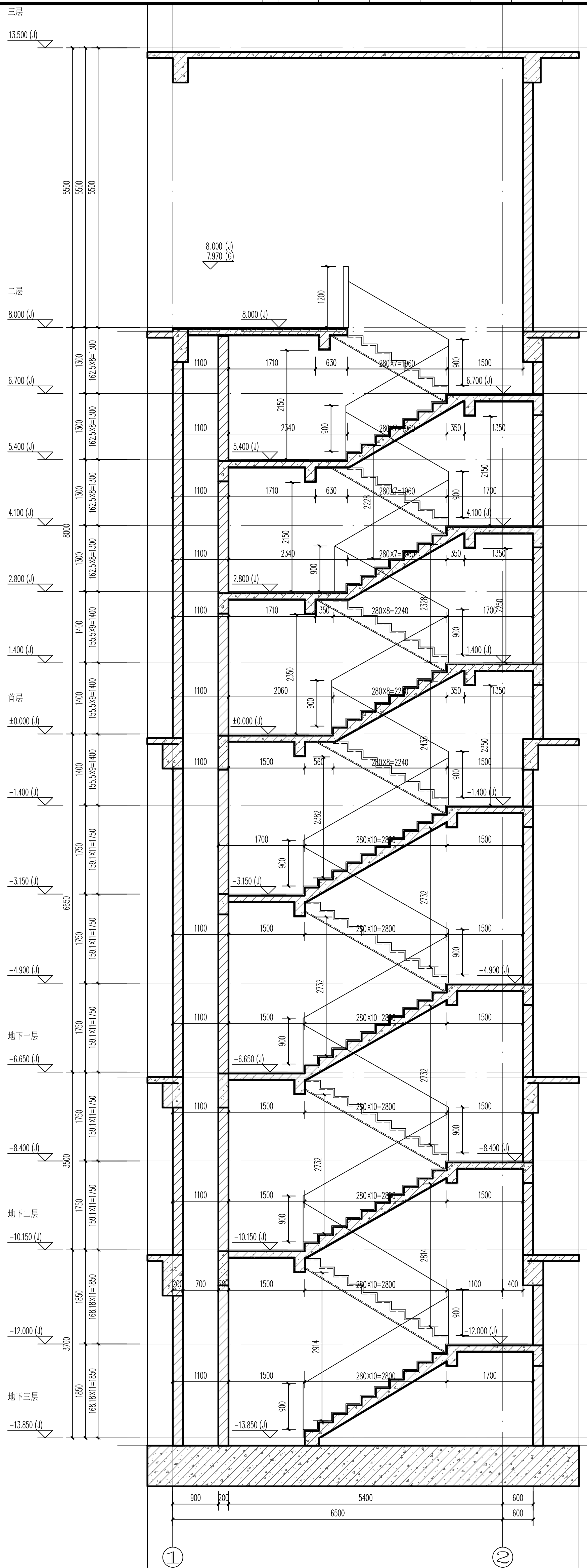
LT05 1-1剖面
