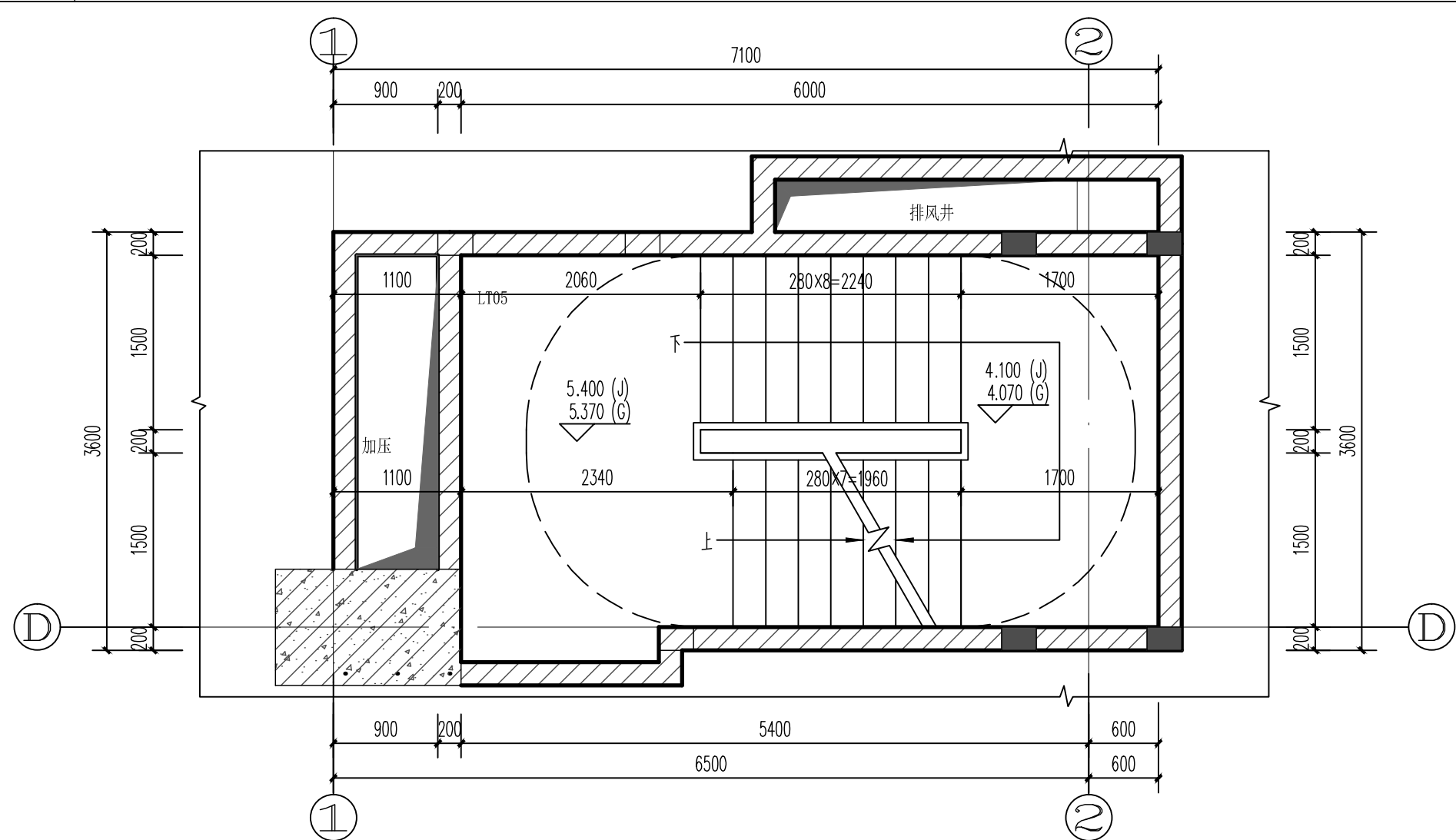
LT05 5.400标高平面
