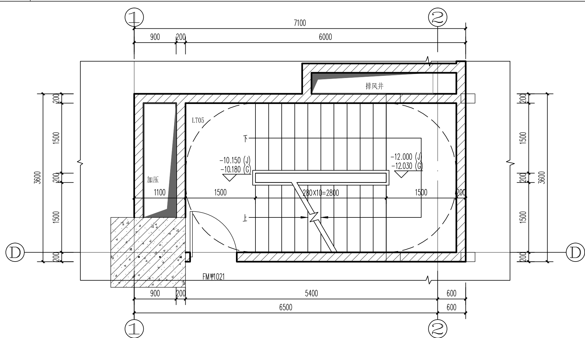
地下二层平面
