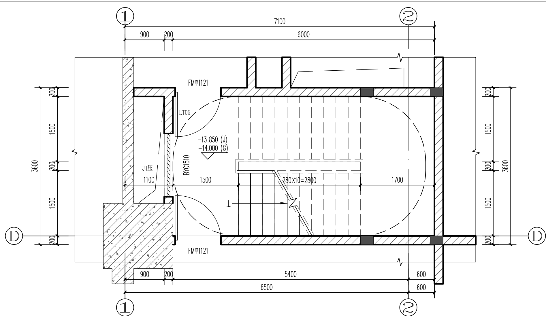
LT05 地下三层平面
