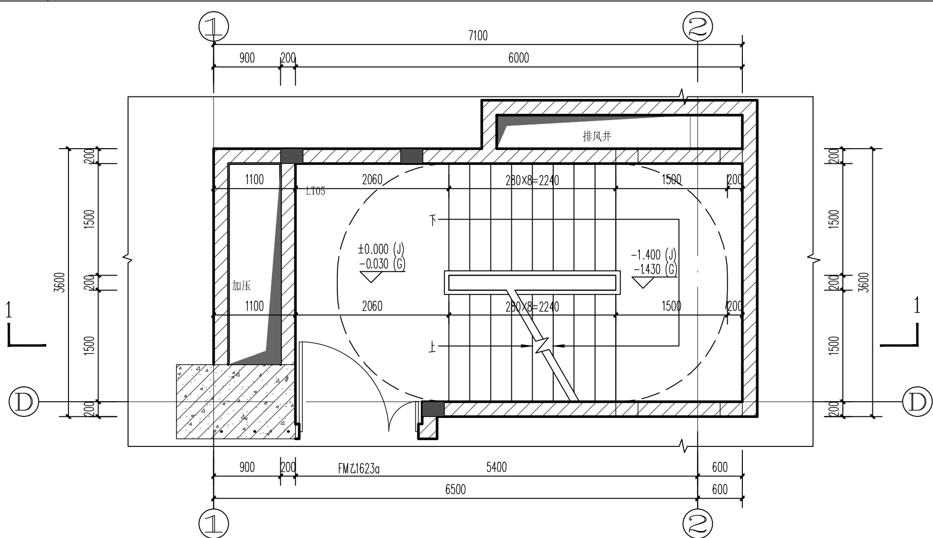
LT05 首层平面
