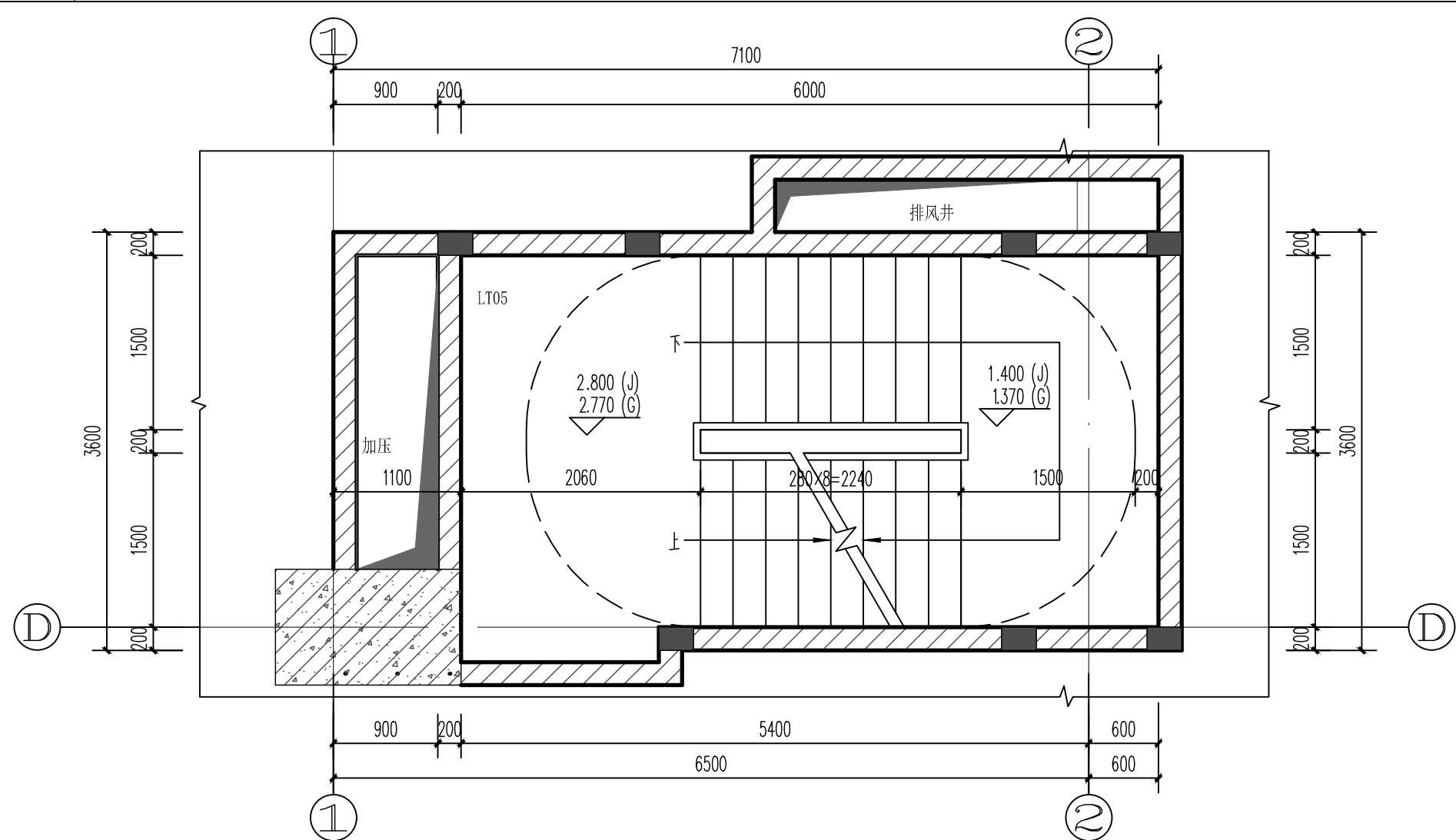
LT05 2.800标高平面
